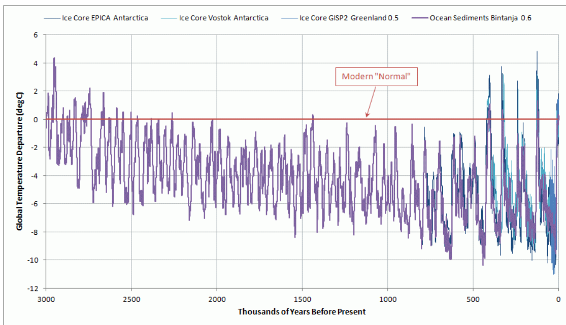
Abbildung 3: Globale Temperatur der letzten drei Millionen Jahre (4)
